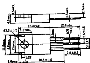
(JEDEC TO-220AB)
